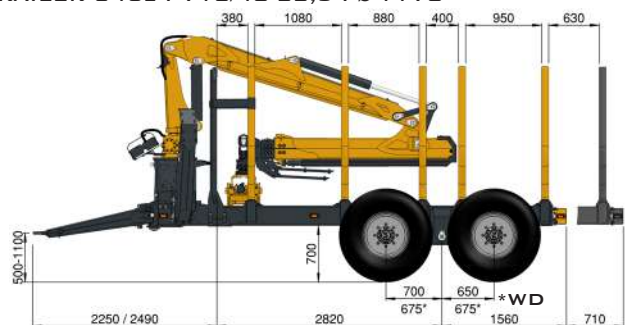
TRAILER 346RE I 710/40-22,5 I Ø 1170
