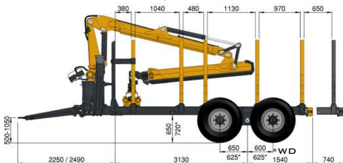
TRAILER 242R | FW | 550/45-22,5 | Ø 1070
