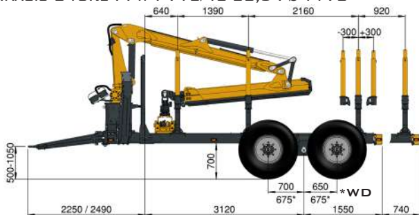
HAAGIS 246RE | FW | 710/40-22,5 | Ø 1170
