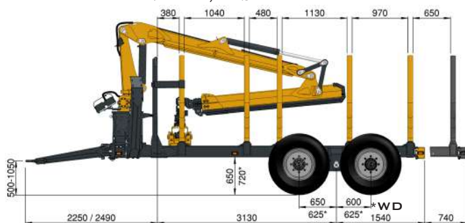
HAAGIS 242R | FW | 550/45-22,5 | Ø 1070
