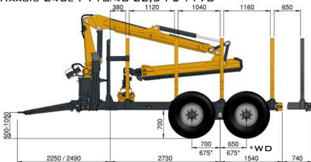
HAAGIS 246E I 710/40-22,5 I Ø 1170
