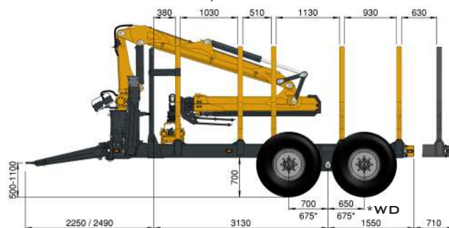
HAAGIS 346E | 710/40-22,5 | Ø 1170
