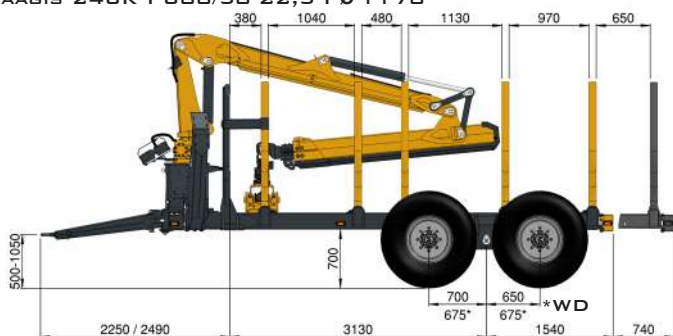
HAAGIS 246R I FW I 600/50-22,5 I Ø 1170
