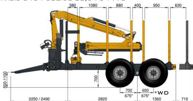
HAAGIS 346R | 600/50-22,5 | Ø 1170
