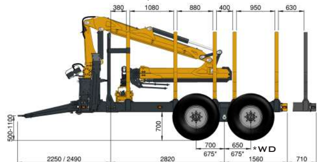
HAAGIS 346RE | 710/40-22,5 | Ø 1170
