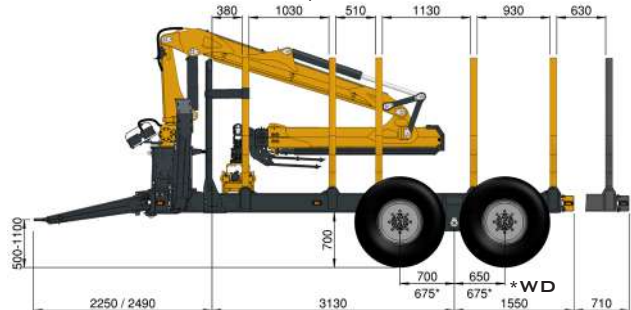
HAAGIS 346RE | 710/40-22,5 | Ø 1170
