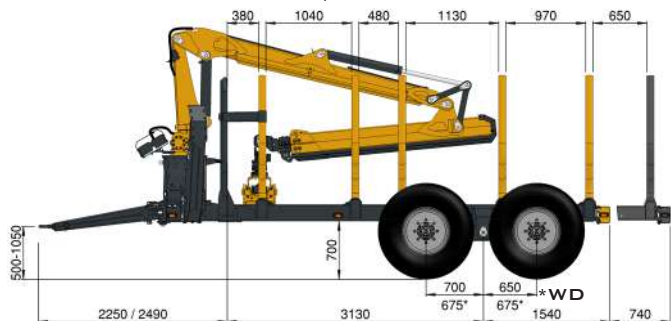
HAAGIS 246RE | 710/40-22,5 | Ø 1170
