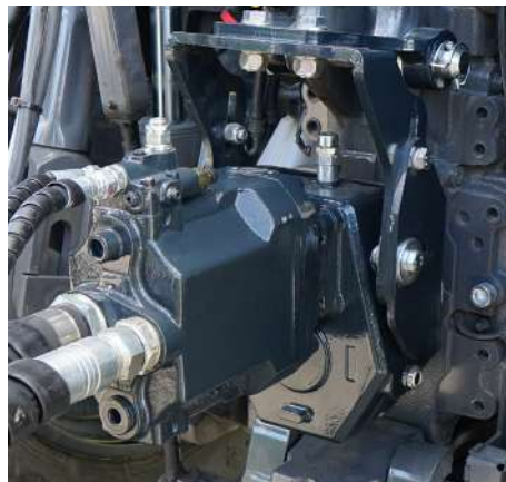
Pump ja reductor PTOs
