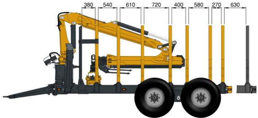
HAAGIS 342R / 346R PIKENDATUD RAAM TIHEDA POSTIJAOTUSEGA
